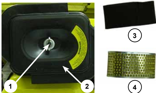
1. Барашковая гайка 2. Крышка фильтра 3. Поролоновый фильтр 4. Бумажный фильтр
